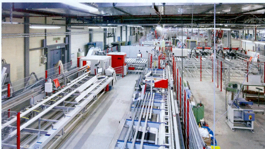
Blick auf das Stabbearbeitungs- zentrum zur Komplettbearbeitung von Fenster- und Haustürprofilen
