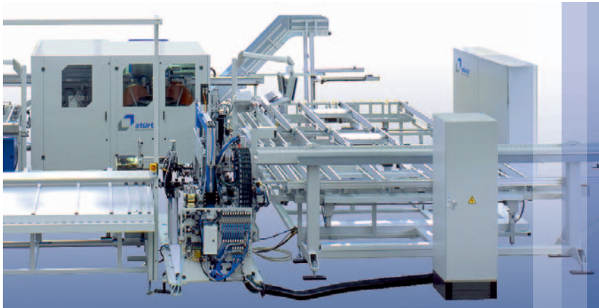
Anlagekonfiguration U-Form, Rechtsausführung » STBAZ JC-LM-100 mit PowerCut JC-LM-300-X
