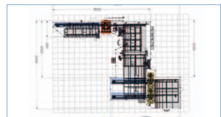
Sonder-Anlagekonfiguration, Rechtsausführung » STBAZ JC-LM-240 mit PowerCut JC-LM-300-X
