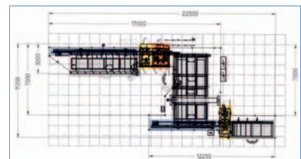
Anlagekonfiguration Z-Form, Rechtsausführung » STBAZ JC-LM-160 mit FlexCut JC-LM-160-X
